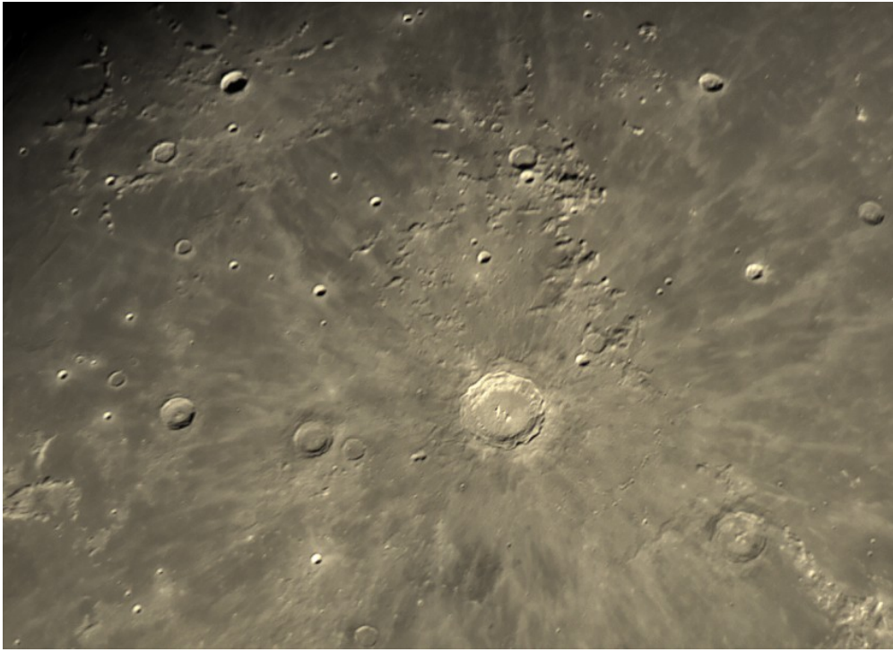
Cratere Copernico - 17/05/2016
