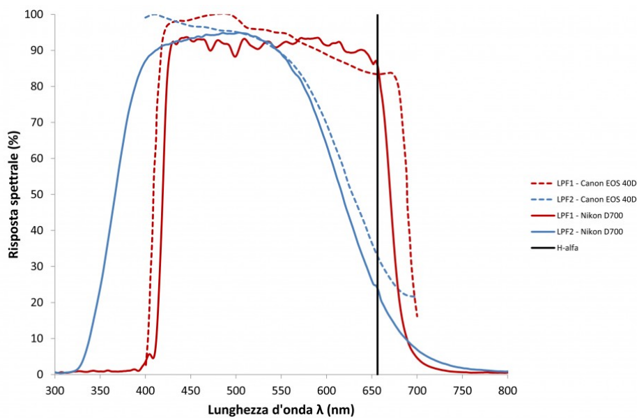
Figura 1: curva di trasmissione per i filtri LPF nel caso delle reflex digitali Canon EOS 40D e Nikon D700
