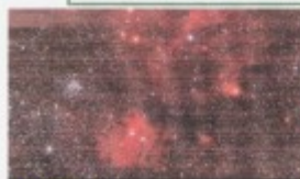
ASTROfisica
