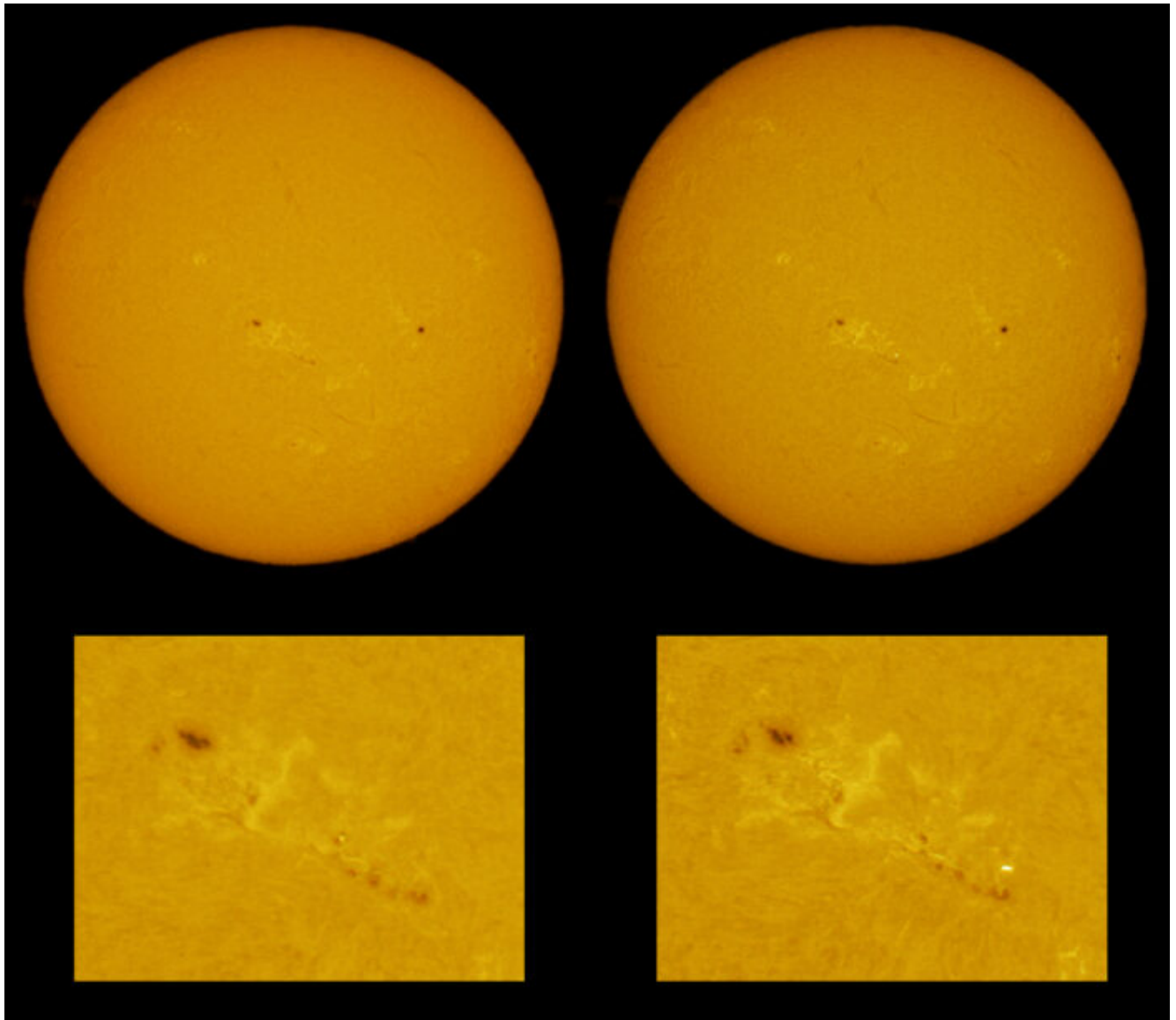
brillamento cromosferico nei pressi della macchia AR4048
