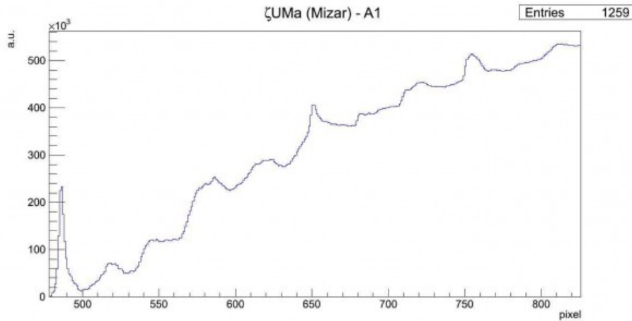
Spettro di ζUMa nella regione compresa tra 500 e 800 pixel
