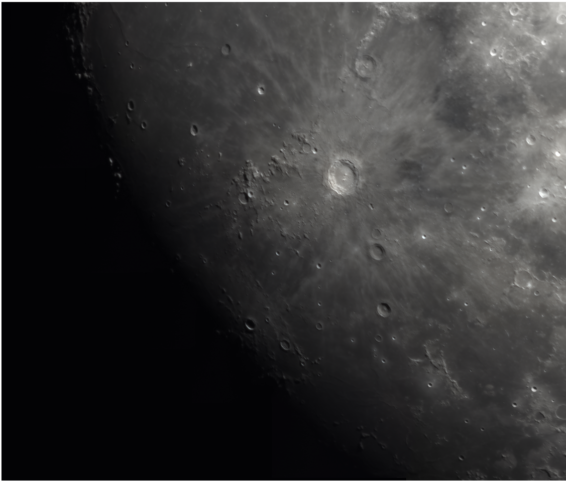
Cratere Copernico - 25/04/2018
