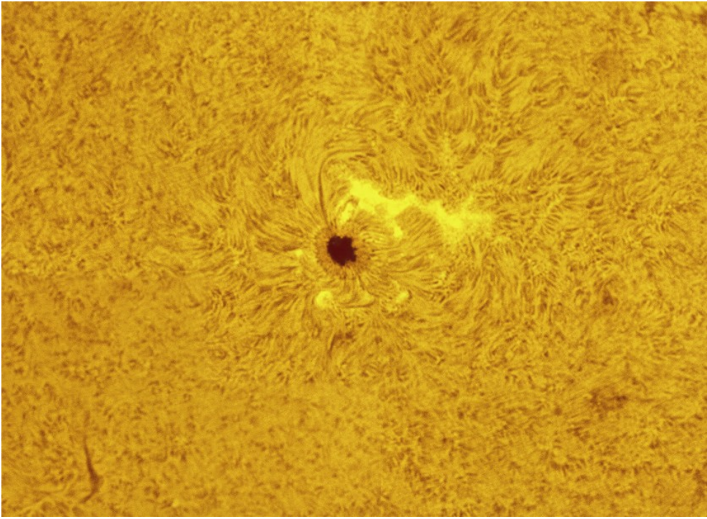
Macchia solare #2546 - 21/05/2016
