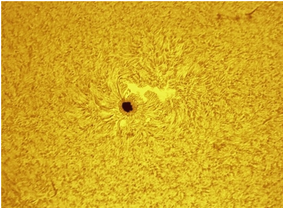
Macchia solare #2546 - 21/05/2016
