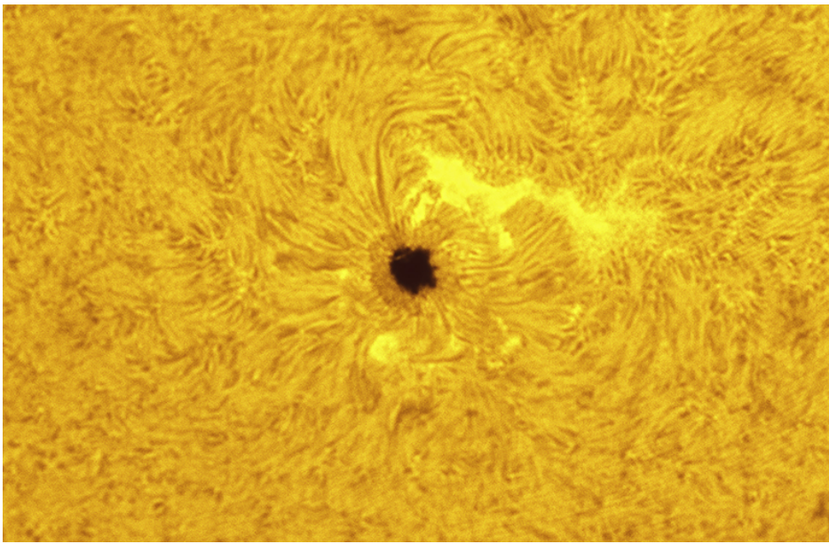
Macchia solare #2546 - 21/05/2016
