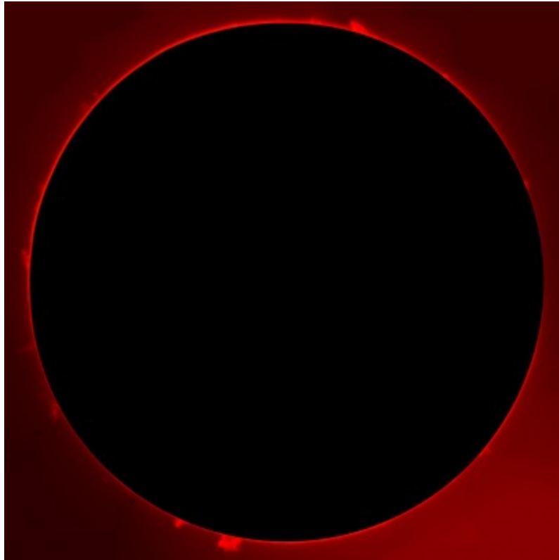
Cromosfera solare - 13/03/2012
