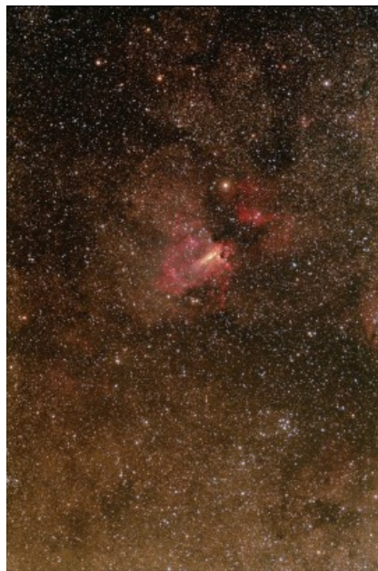
M17 (NGC 6618) - 16/06/2012
