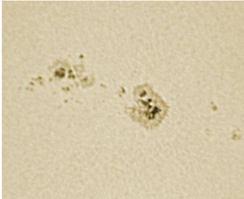
Macchia solare 1054 - 14/03/2010
